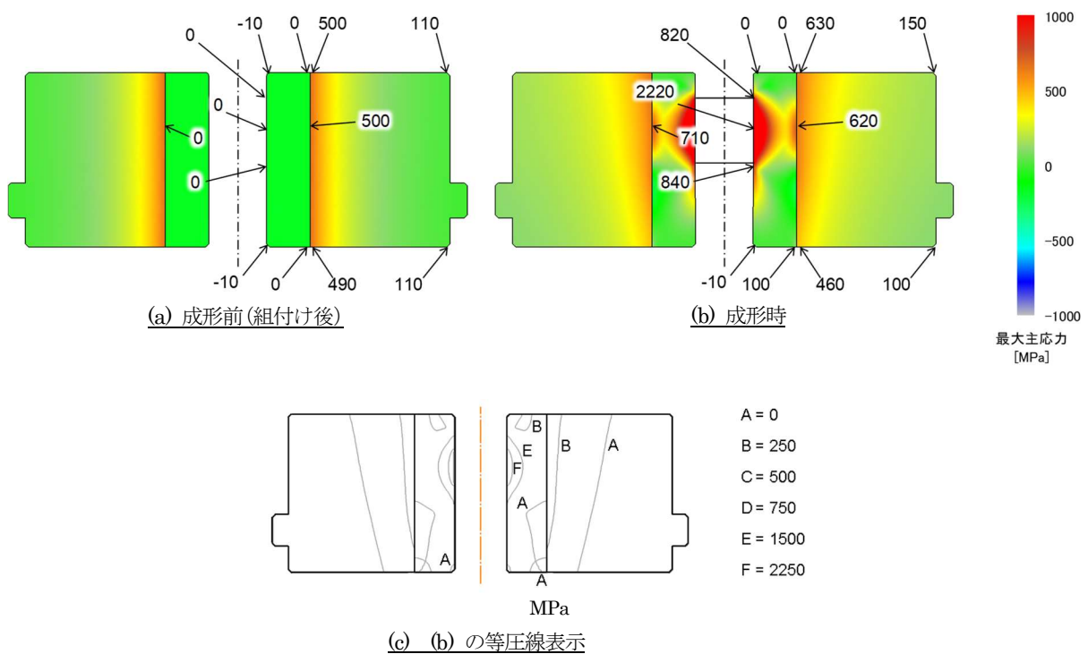
図 9.19 組合せダイスの圧力作用域幅の影響 (株式会社ヤマナカゴーキン提供)
